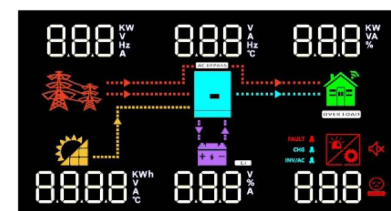
LCD DISPLAY
